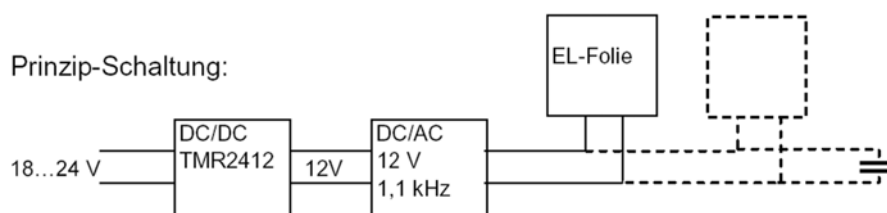
Abbildung 4: Versuchsaufbau
